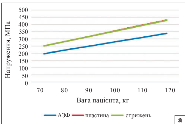
Рис. 10. Графіки залежності величин напружень від ваги пацієнта в елементах металевих конструкцій (а) та навколо фіксуювальних гвинтів і стрижнів (б) у великогомілкової кістки за її перелому у верхній третині та різних видів остеосинтезу
