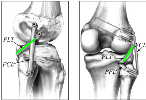
Рис. 2. Реконструкція задньолатерального кута за LaPrade. Вигляд із латерального боку та позаду. FCL — пучок, який відновлює малоюмілку обідну зв'язку, PLT — сухожилок підколінного м'яза, PFL — підколінно-малоюмілку зв'язка [3]
