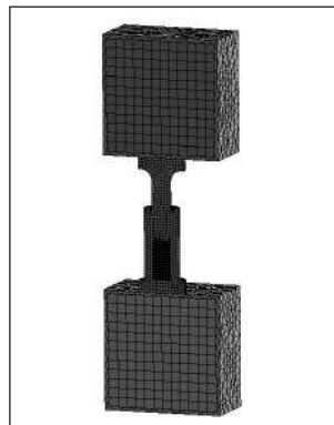
Рис. 4. Скінченно-елемента модель
