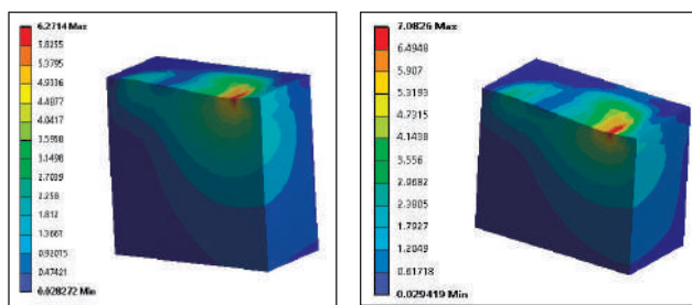
Рис. 23. Еквівалентні напруження в губчастій тканині (нижній елемент)
