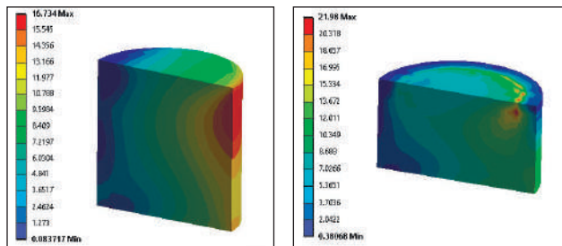
Рис. 19. Еквівалентні напруження в «Елемент-3» ендопротеза
