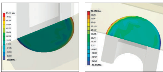
Рис. 26. Контактний тиск у парі «Елемент-2 – Коркова тканина (нижній елемент)»
