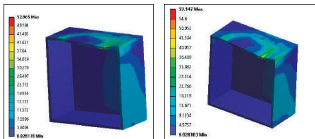
Рис. 21. Еквівалентні напруження в корковій тканині (нижній елемент)
